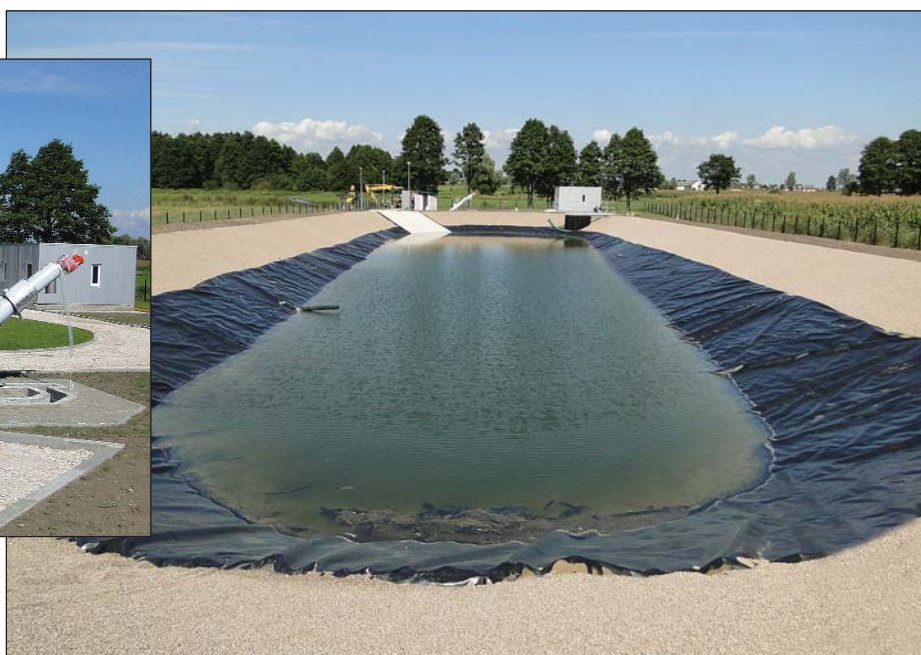
Oczyszczalnia ścieków w Gralewie - gotowa...
