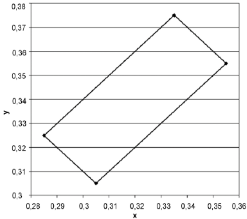
Rys. 1. Współrzędne chromatyczności x,y dla barwy białej oznakowania
